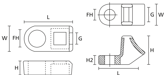
FH Befestigungssockel (Draufsicht und Seitenansicht)
