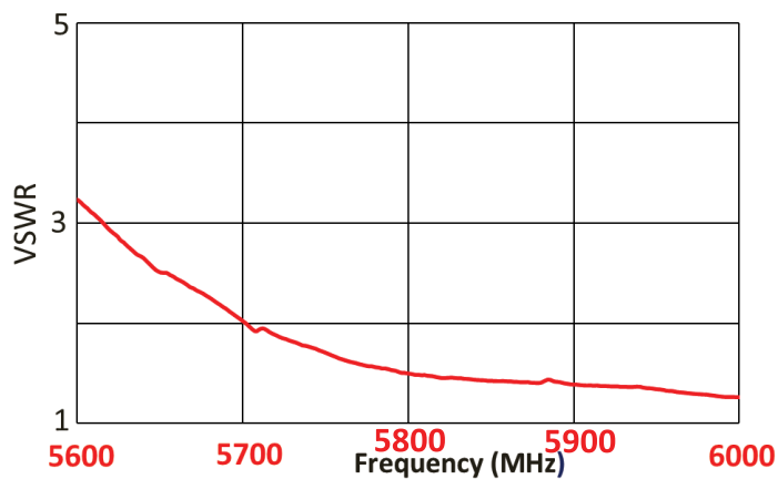
VSWR
