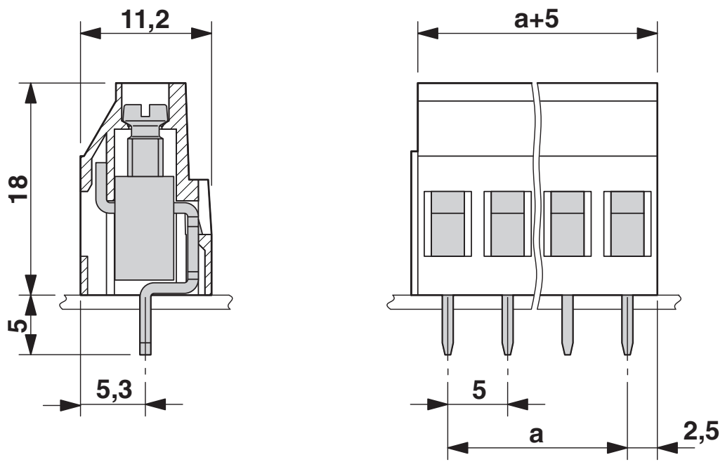
尺寸图
