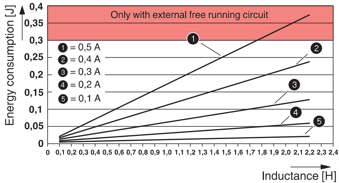
电感负载断开时的最大输出能耗
