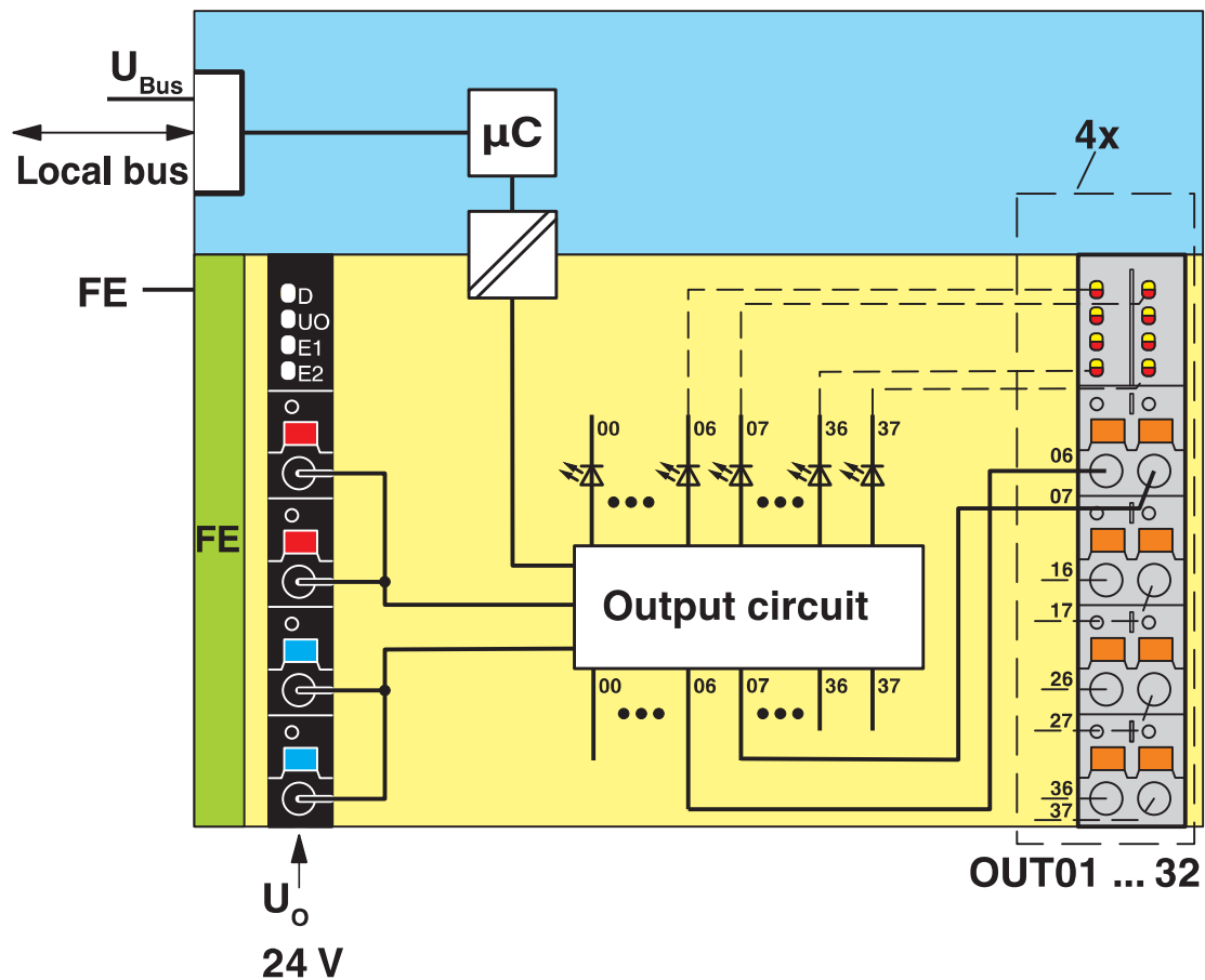
结构框图
