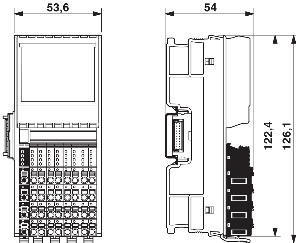
尺寸图
