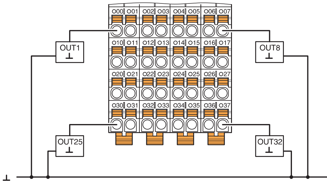
接线图
