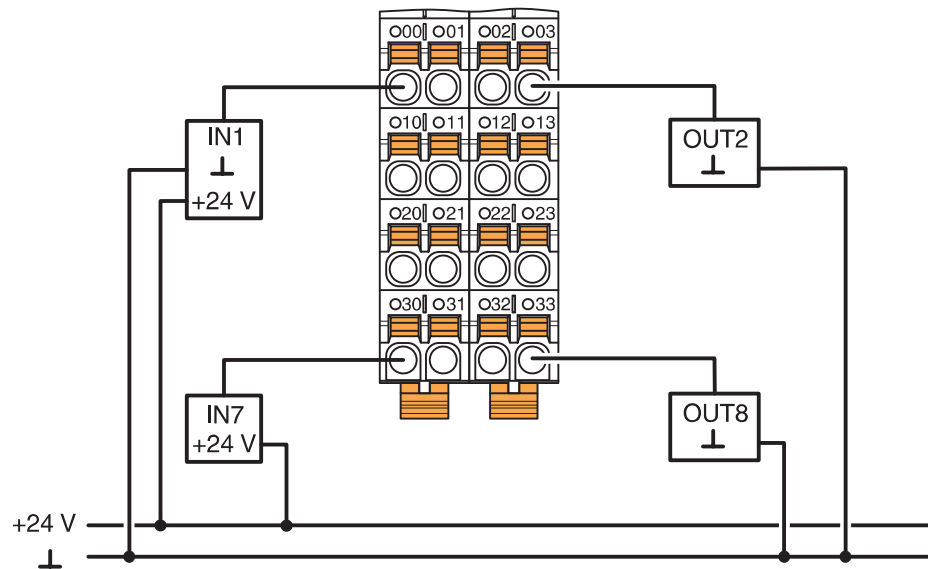
接线图
