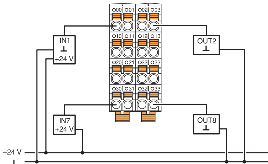
接线图
