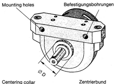
Centering collar / Zentrierbund
