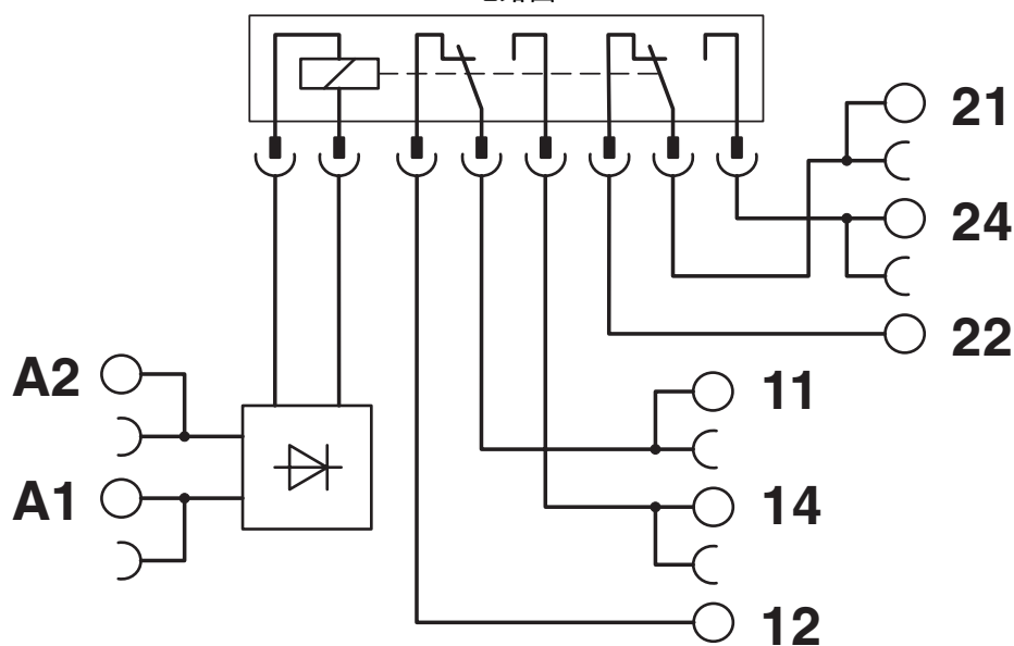
电路图
