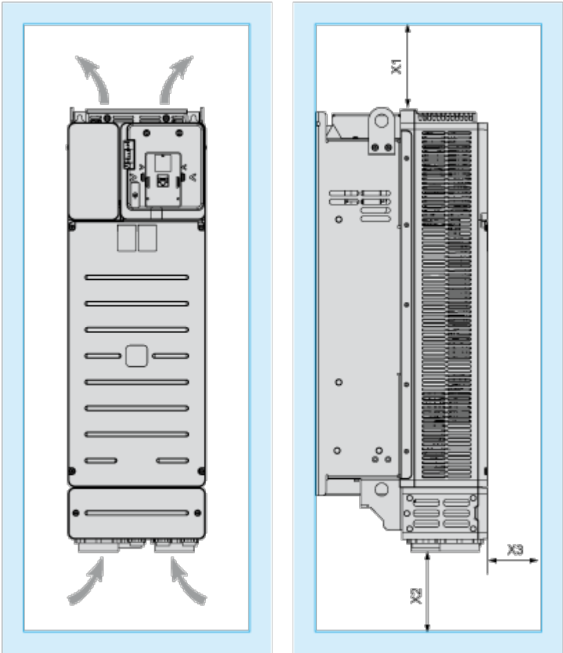
尺寸 (毫米)
