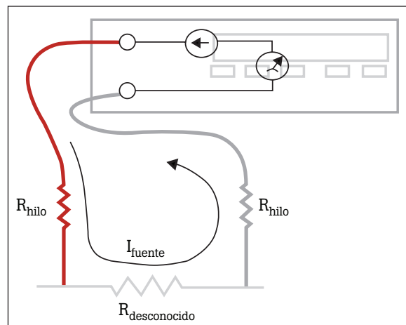
Figura 1: las medidas de resistencia con dos hilos inducen a error debido a las caídas de tensión en los cables de prueba.
