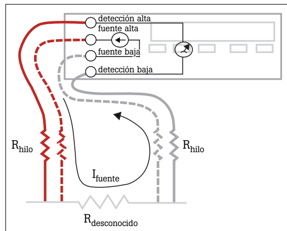
Figura 2: las medidas de resistencia con cuatro hilos eliminan la corriente en los hilos de tensión y, por tanto, esta posible fuente de errores.
