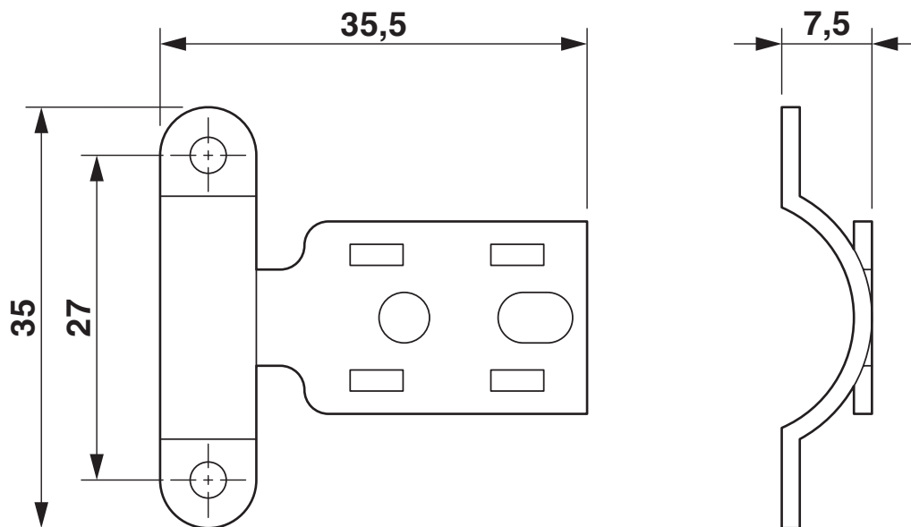
尺寸图
