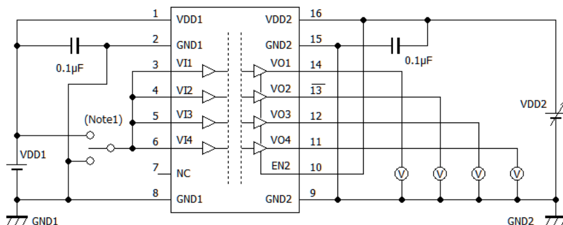
Fig.12-1-4. DCL540C01/DCL540D01 VDD2 UV+ / VDD2 UV Test Circuit
