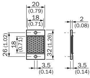
尺寸图 (尺寸单位: mm)
