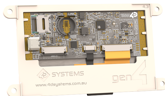
gen4-ESP32-43CT Rear
