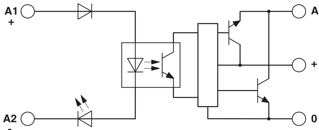
Schaltplan
