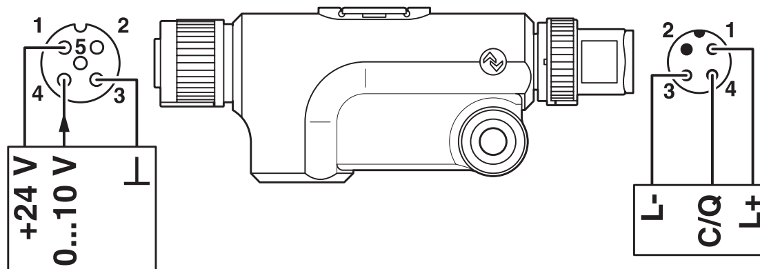
接线图
