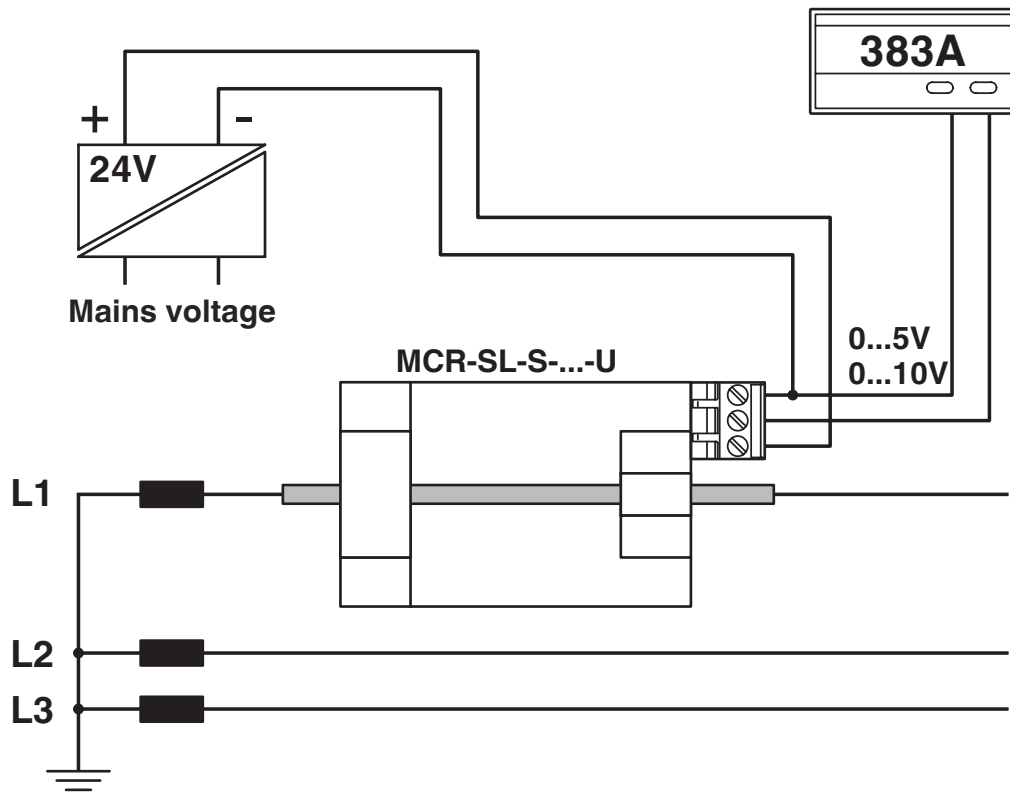
Applikationszeichnung
