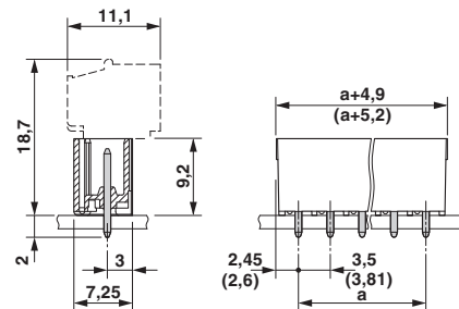
外形寸法
