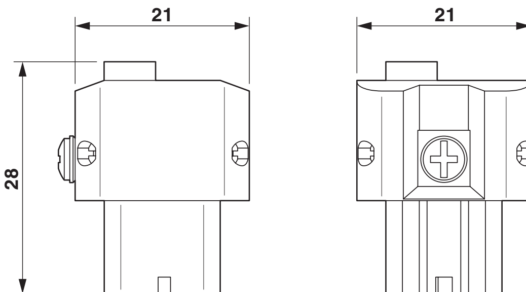
Maßzeichnung
