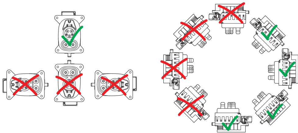
接线图
