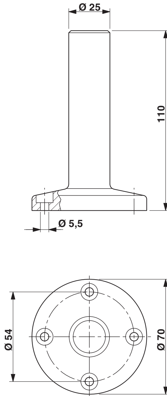
尺寸图
