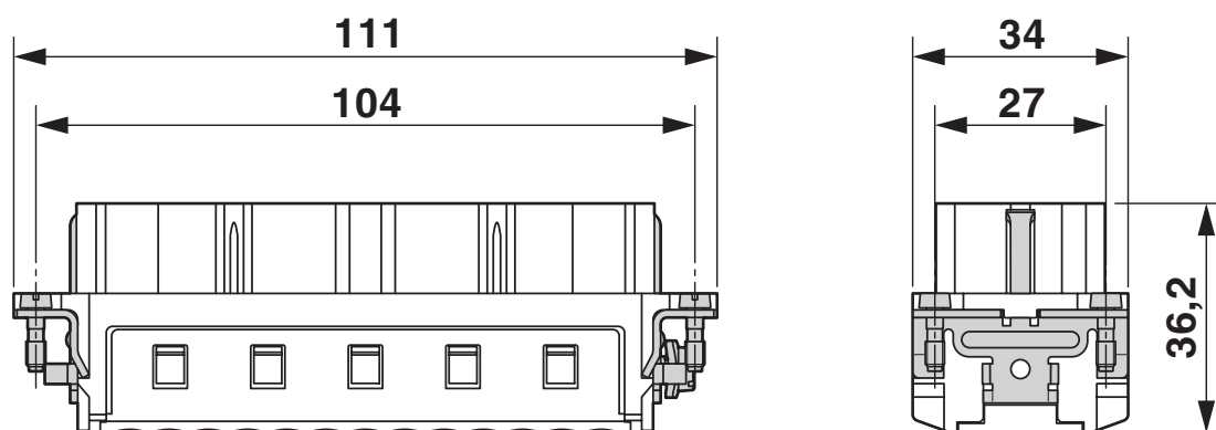
尺寸图
