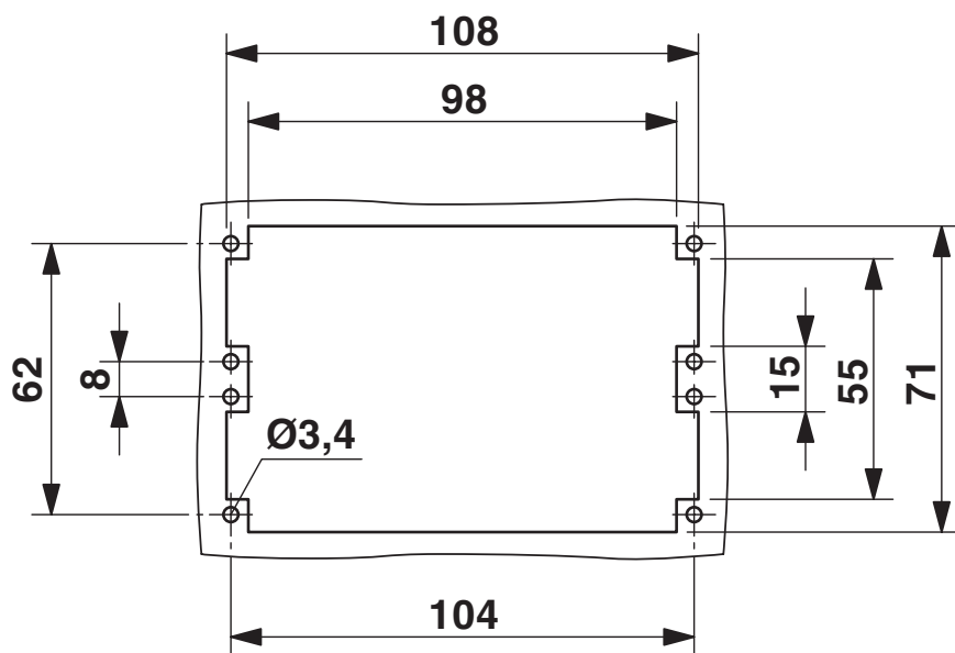
尺寸图
