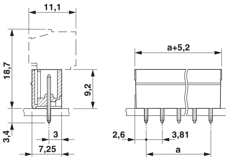
尺寸图
