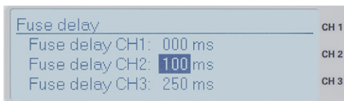
Abb. 5.3: Einstellung der Fuse Delay (R&S®HMP2030)
