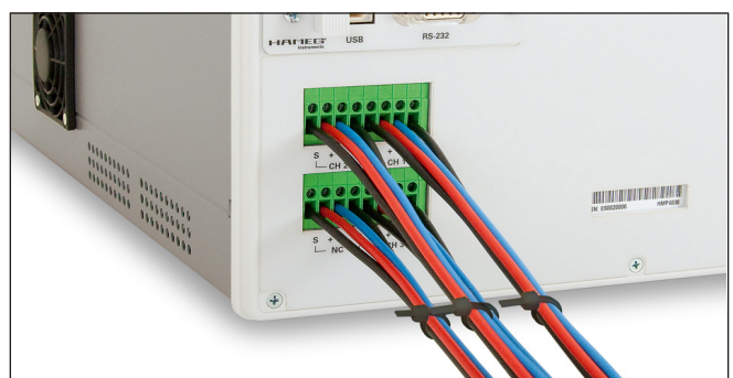
Abb. 3.4: R&S®HMP4040 Anschlussleisten auf der Geräterückseite
