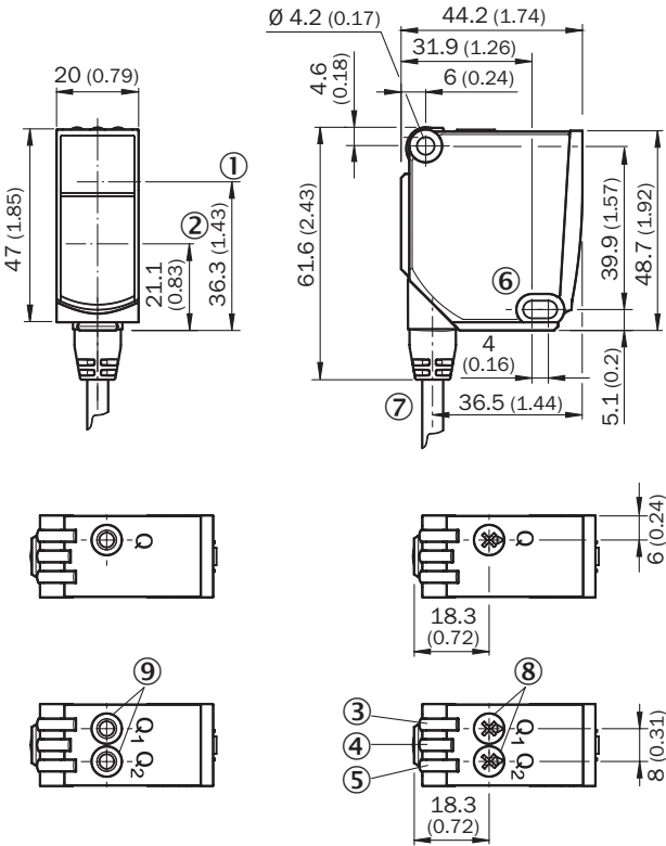
尺寸图 (尺寸单位: mm)
