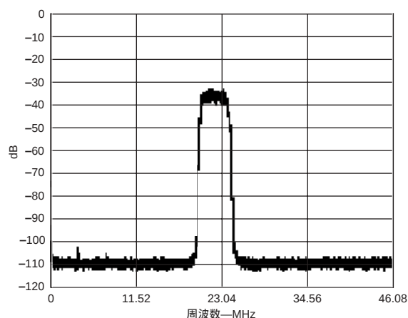
特性32 FFT : f_s = 92.16\text{MSPS} , f_{IN} = 70.3\text{MHz} , WCDMA @ 70.0MHz、SFDRをイネーブル
