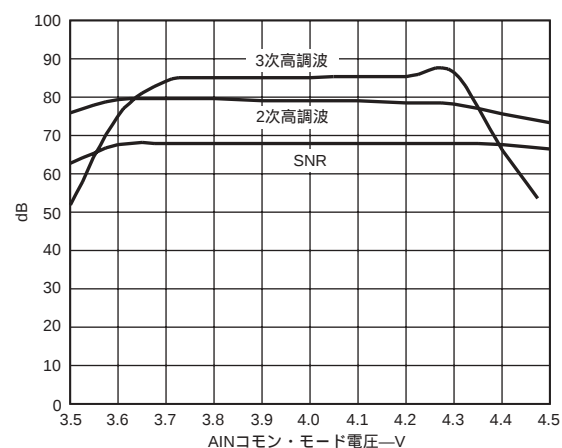
特性11 ダイナミック性能 対 AINコモン・モード電圧差動 AIN@ -0.5dBFS、 f_{IN} = 49.3\text{MHz} 、 f_s = 105\text{MSPS}
