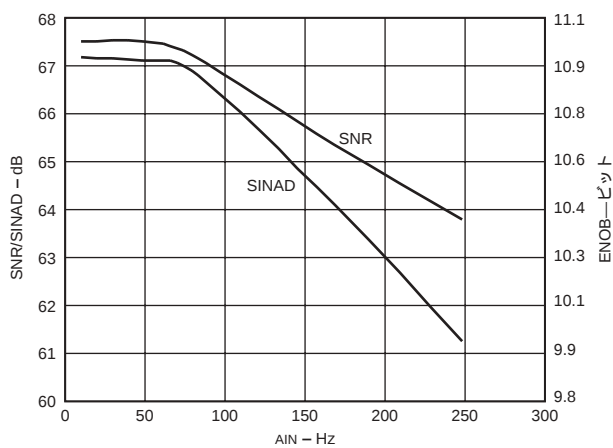
特性5 S/N比対AIN周波数差動AIN @ -0.5dBFS、 105MSPS、SFDRをディスエーブル
