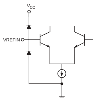
図6 リファレンス入力
