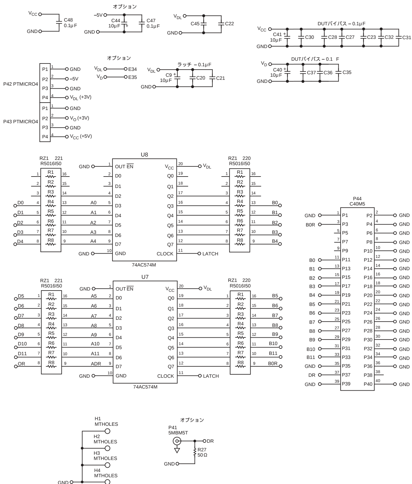
図15 評価ボードの回路図
