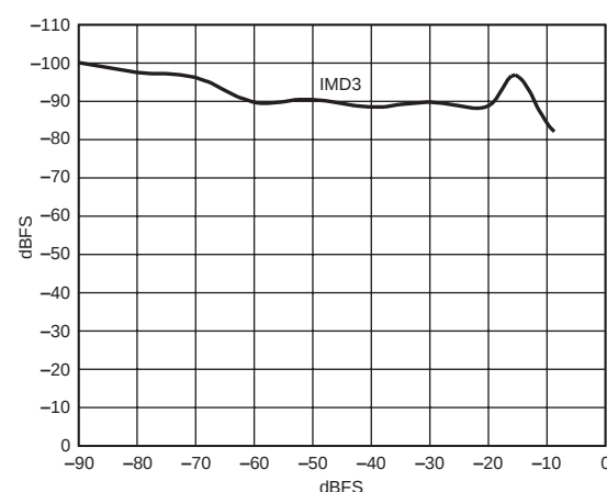
特性30 3次IMD 対 AINレベル、 f_s = 105\text{MSPS} 、 f_{IN} = 150.3 および 151.3\text{MHz} 、差動AIN、SFDRをイネーブル
