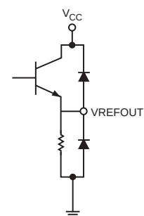
図4 リファレンス出力
