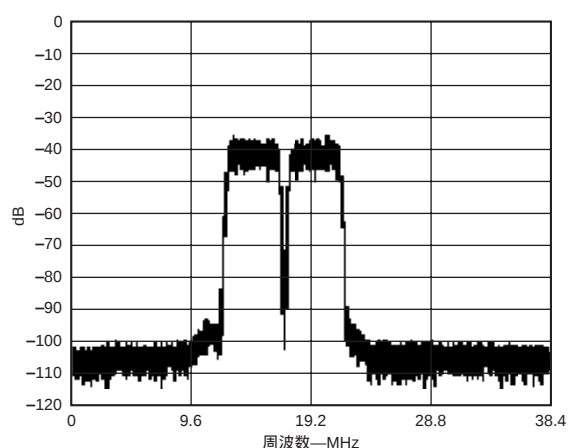
特性31 FFT : f_s = 76.8\text{MSPS} , f_{IN} = 59.6\text{MHz} , 2種のWCDMAキャリア、差動AIN、SFDRをイネーブル
