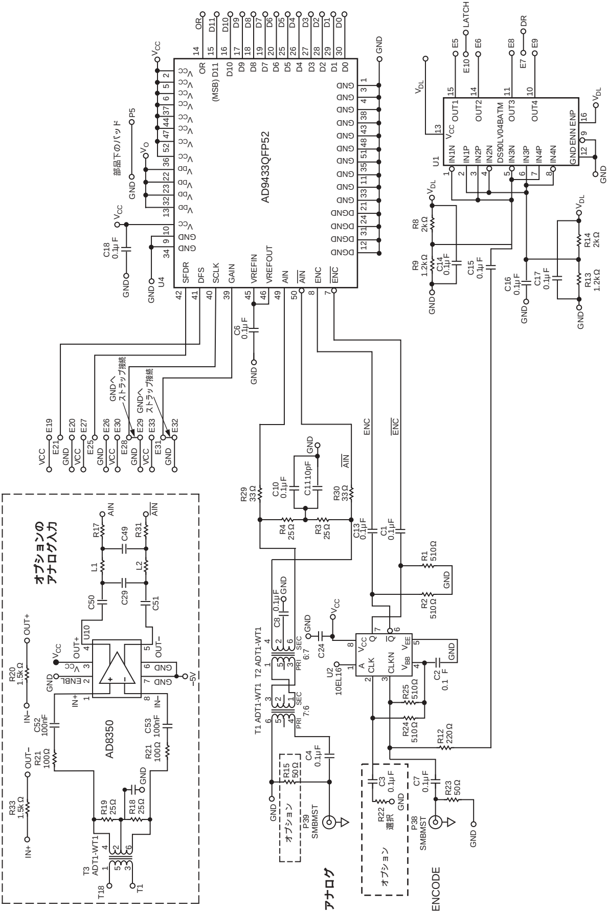
図13 評価ボードの回路図
