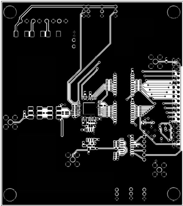
図17 表面配線
