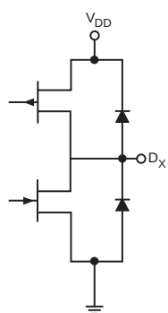
図2 デジタル出力
