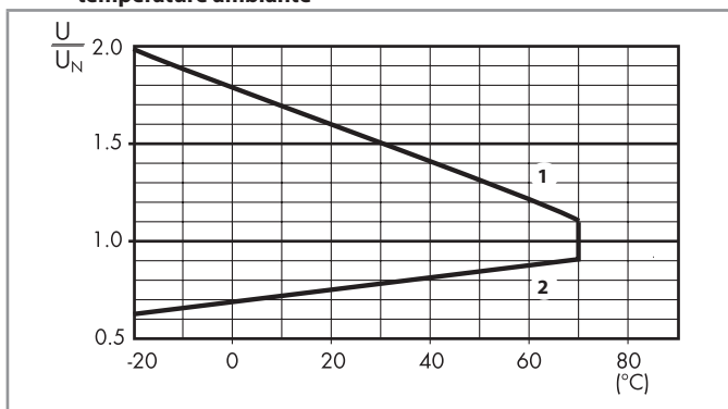
R 46 - Plage de fonctionnement bobine DC en fonction de la température ambiante
