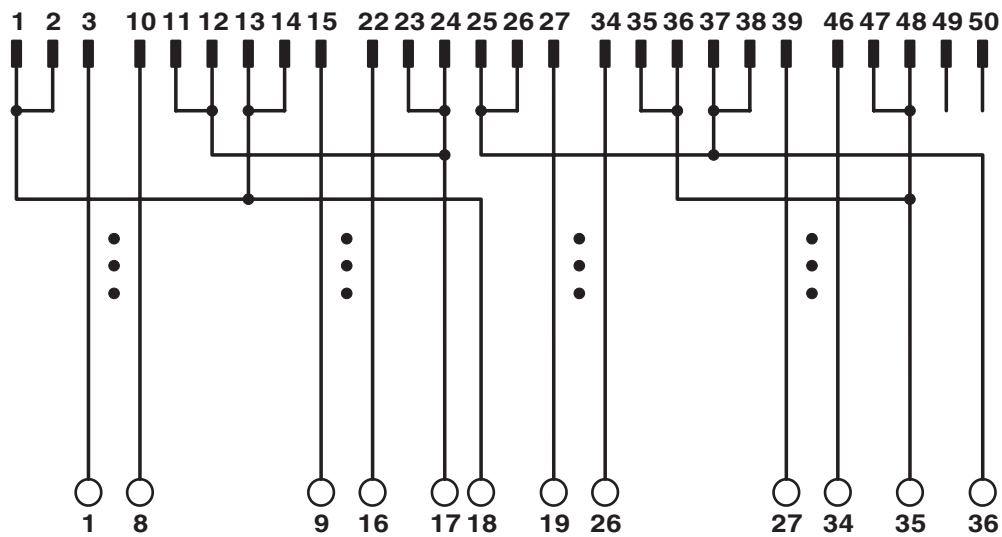
Anschlussbild VIP-2/.../FLK50/AB-1756
