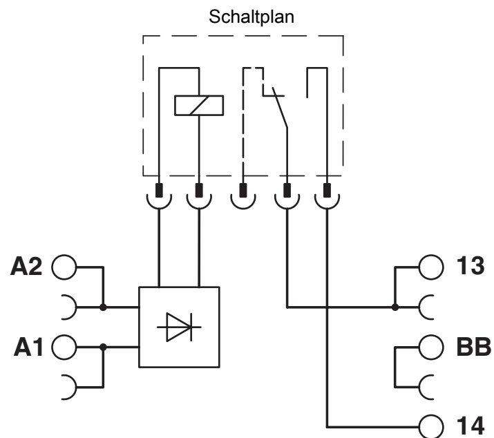
Schaltplan
