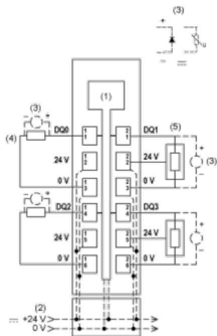
接线图
