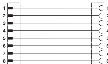
回路図
