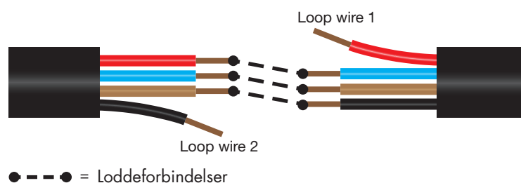
Montage af flerleder kabel
