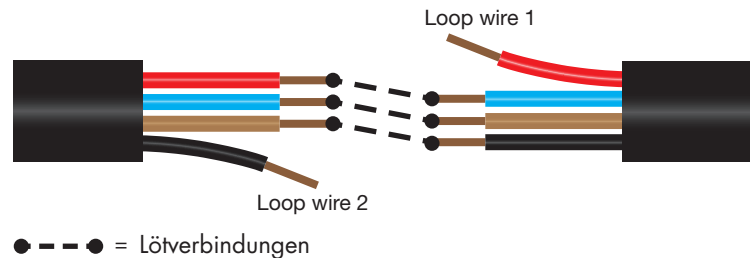
Lötanleitung für Kabel mit mehreren Leitern
