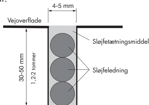
Sløjfe med flere viklinger
