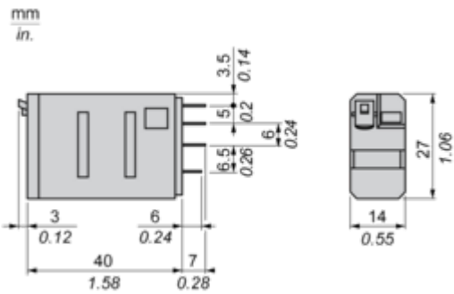
Stecker-Seitenansicht
