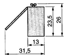
Pièce d'adaptation pour renvoi à 90° XUP-Z01
