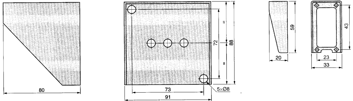
Boîtier de protection pour réflecteur XUZ-C80 XUZ-D15
