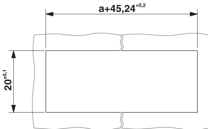
Maßzeichnung
