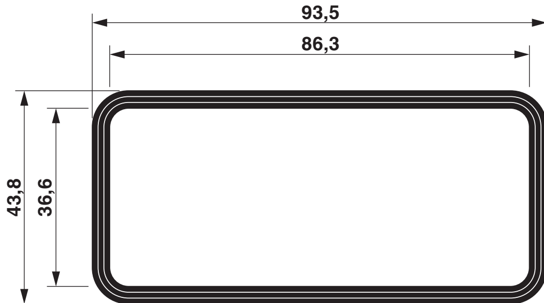
尺寸图
