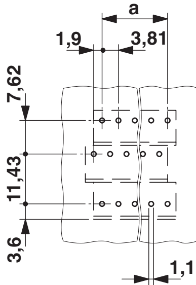
开孔图/焊盘环宽
