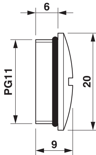
尺寸图
