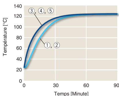
Distribution de la température de 120 °C
