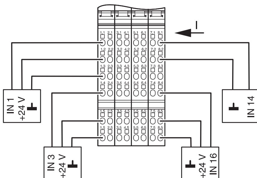
接线图
