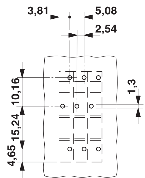
开孔图/焊盘环宽
