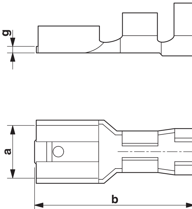
Maßzeichnung
