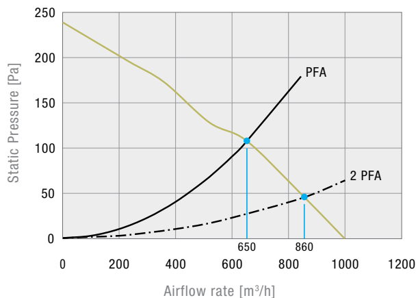
PTF 61.000 IP 33
