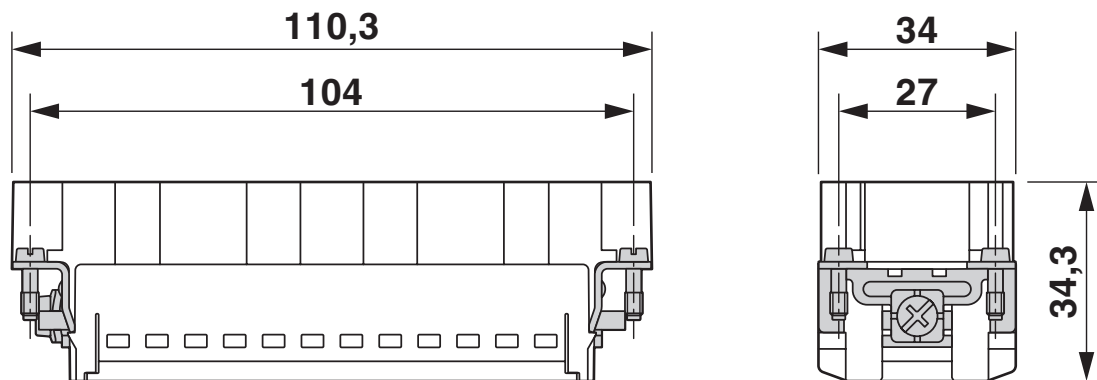
尺寸图
