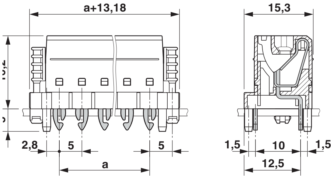
尺寸图
