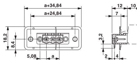
外形寸法
