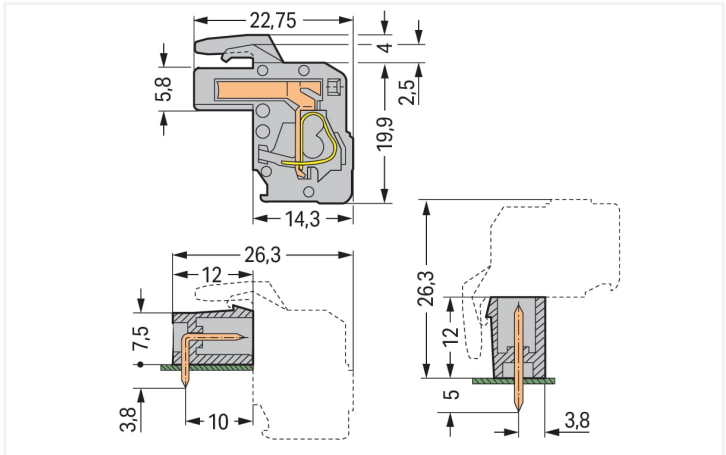
Dimensions en mm L = (\text{nombre de pôles} \times \text{pas}) + 1,5 \text{ mm} + 0,9 \text{ mm} Connecteurs femelles de 2 à 3 pôles – seulement 1 crochet d'arrêt
