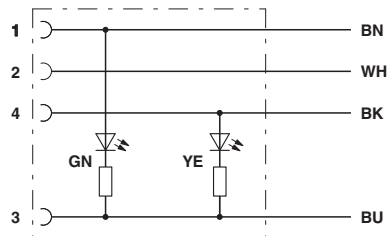
回路図
