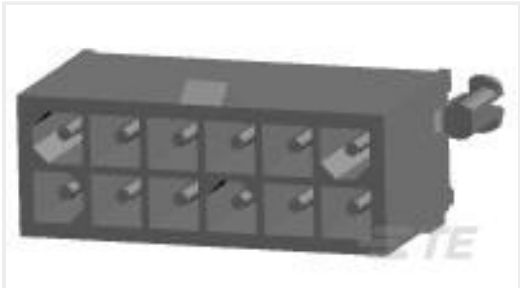
TE Part #1-794066-0 12P MINI UMNL HDR W/DH SN LF
