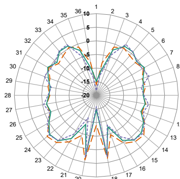
YZ-Plane Gain
