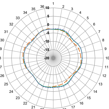
XZ-Plane Gain
