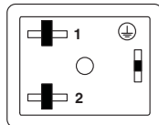
配線図
