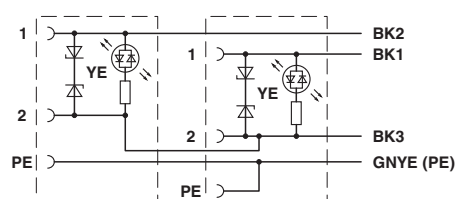
回路図
